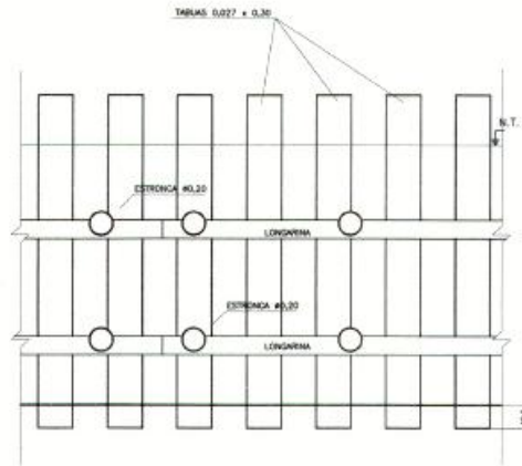
ELEVACAO
