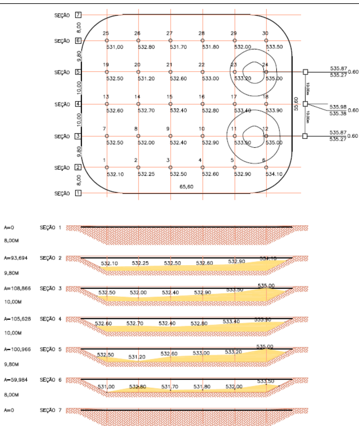
Figura 6. Cálculo dos volumes do Lodo na Lagoa Anaeróbia.
