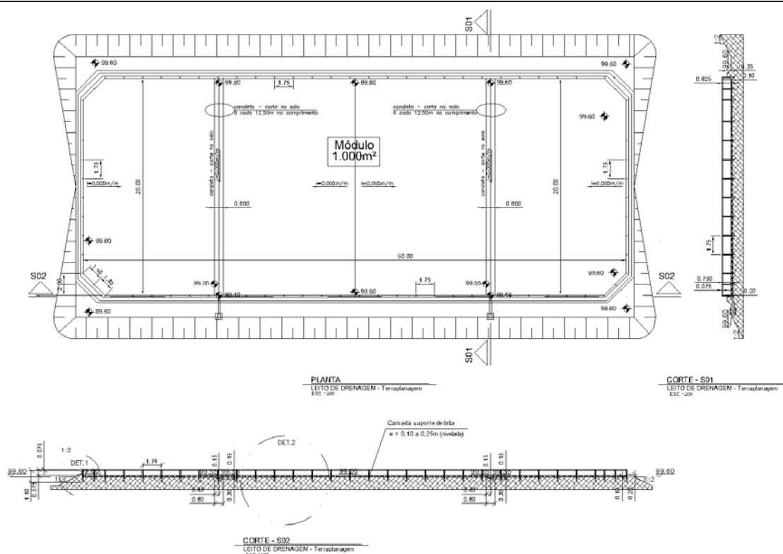
Figura 7. Leito de Drenagem – Módulo 1000m 2
