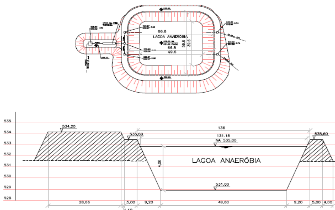
Figura 4. ETE.2 – Lagoa Anaeróbia
